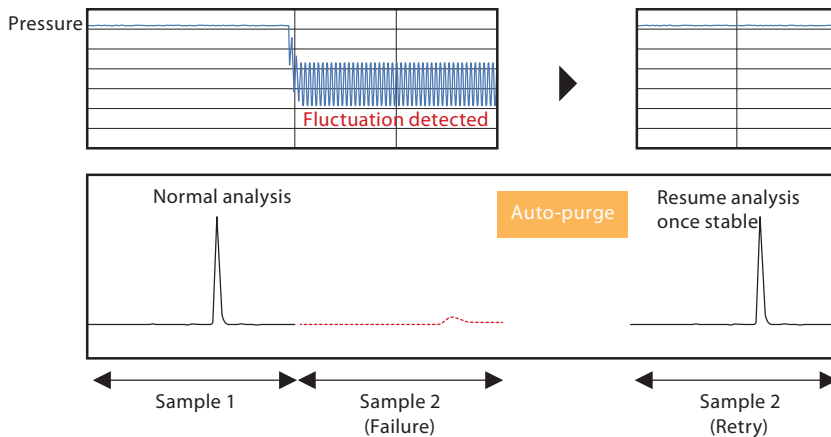
Рисунок 6. Автоматическое восстановление нормальной работы системы в случае попадания пузырьков воздуха в линию подачи подвижной фазы
