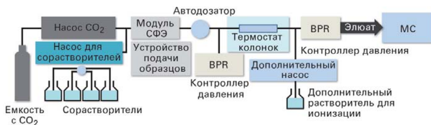
Рисунок 1: Конфигурация системы Nexera UC SFE-SFC-MS
