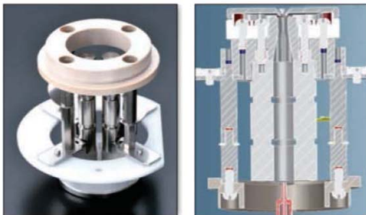
Рисунок 11. Система ионной оптики UF Qarray, обеспечивающая высочайшую чувствительность LCMS-8060
