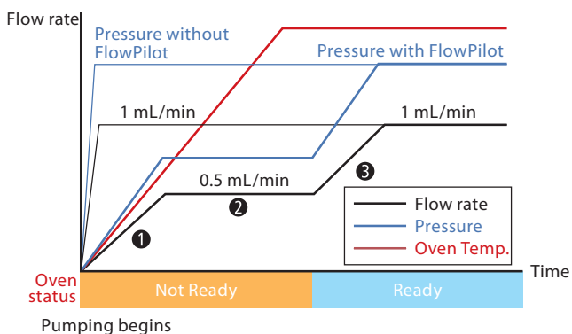
Рисунок 5. Предотвращение скачков давления подвижной фазы при помощи функции Smart Flow Pilot
