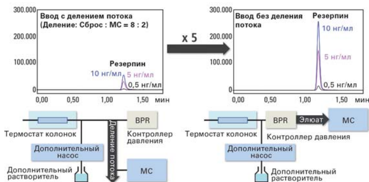
Рисунок 4: Увеличение чувствительности анализа благодаря использованию контроллера давления с минимальным мёртвым объёмом
