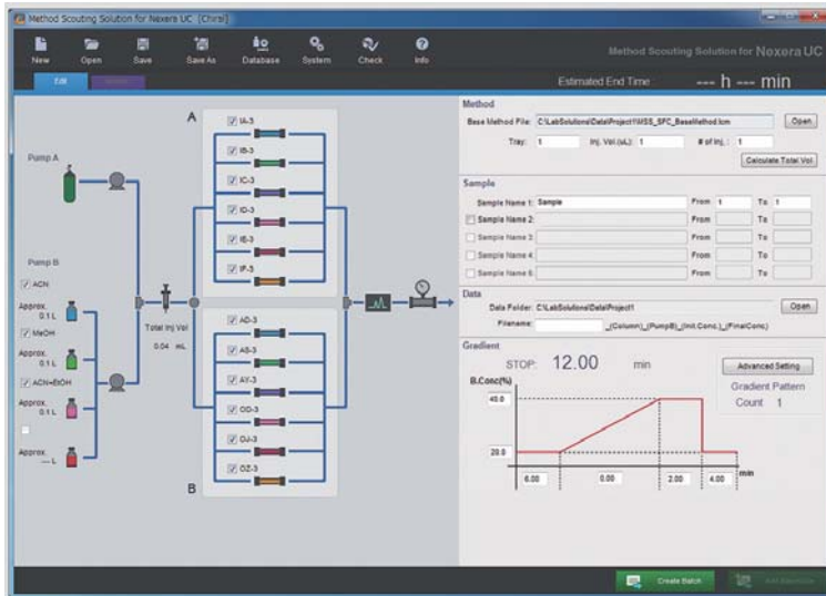
Рисунок 3: Программа «Method Scouting Solution», окно программирования условий анализа
